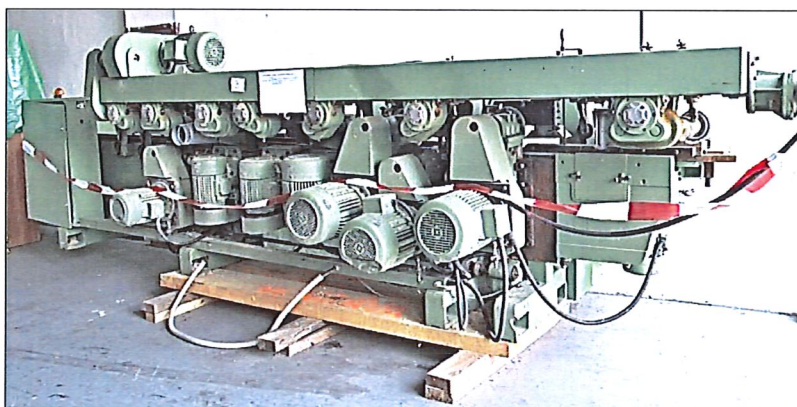
Obrázek 3 – Čtyřstranná frézka
