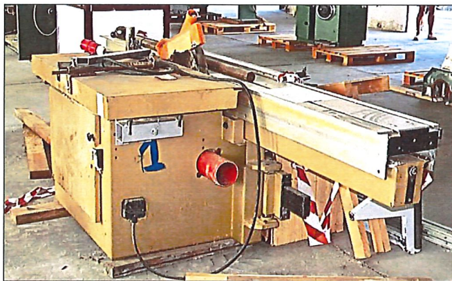
Obrázek 6 – Spodní okružní pila s pojezdovým stolem SCM
