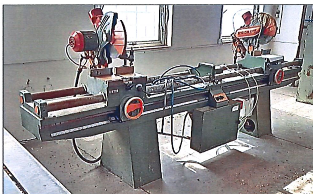
Obrázek 21 – Dvoukotoučová radiální zakracovací a pokosová pila OMS SALVARANI
