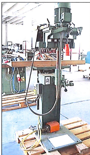
Obrázek 13 – Třívřetenová stojanová vrtačka REICHENBACHER
