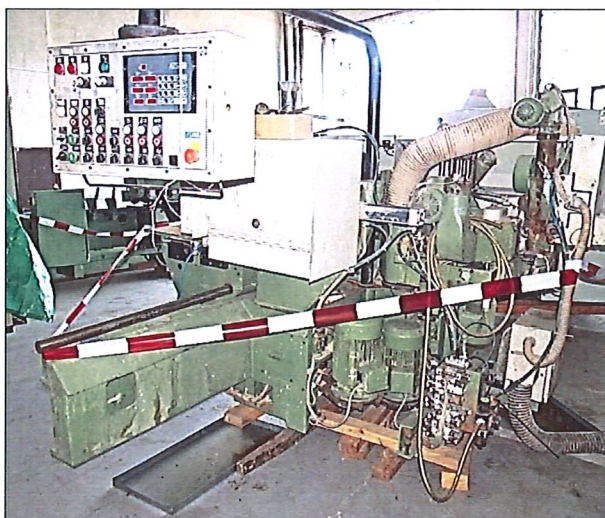
Obrázek 1 – Čepovací – profilovací stroj UNICONTROL 5
