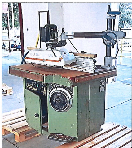
Obrázek 16 – Spodní frézka s horním podavačem
