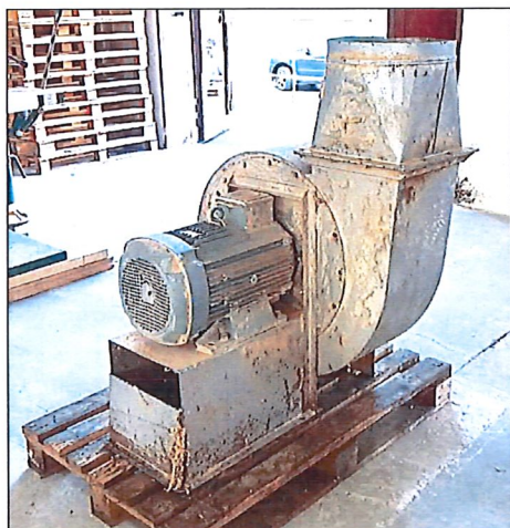
Obrázek 24 – Ventilátor odsávání s motorem GRUSS
